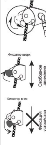
Рис. 7. Положение фиксатора
