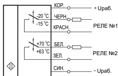
Схема подключения
