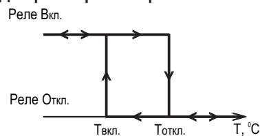
Диаграмма работы реле №2
