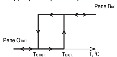
Диаграмма работы реле №1
