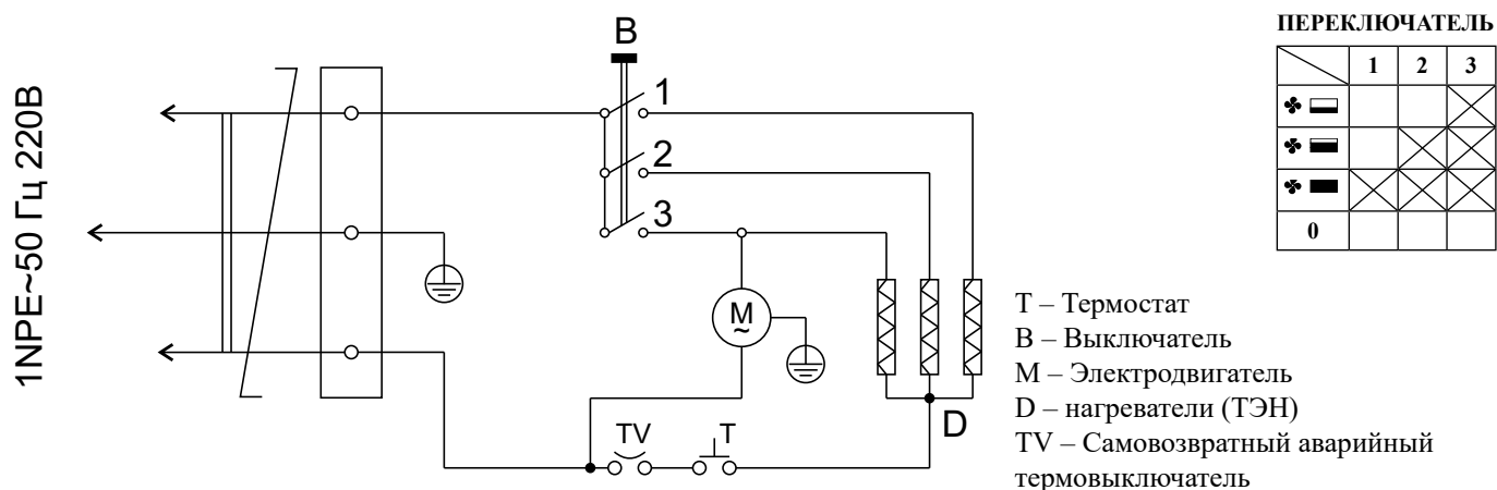
Рисунок 5. Электрическая схема тепловентилятора КЭВ-2С41Е
