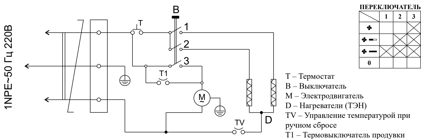
Рисунок 6. Электрическая схема тепловентилятора КЭВ-3С41Е
