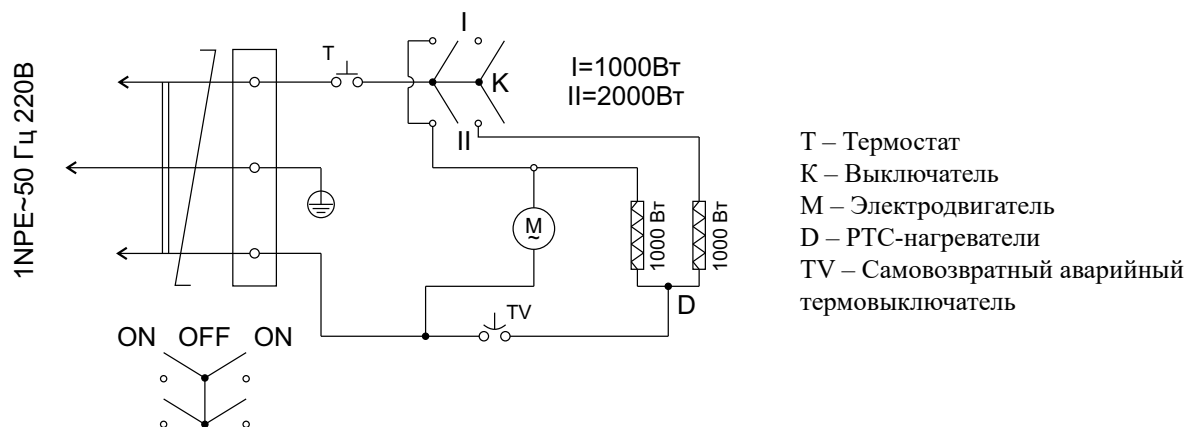
Рисунок 2. Электрическая схема тепловентилятора КЭВ-2С51Е
