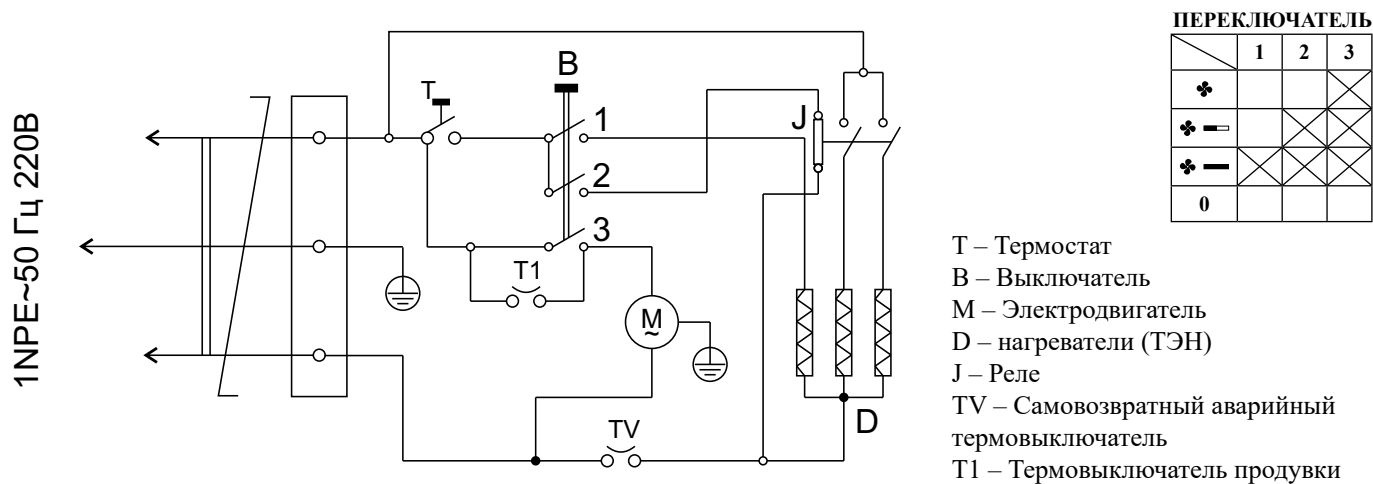
Рисунок 7. Электрическая схема тепловентилятора КЭВ-4С41Е
