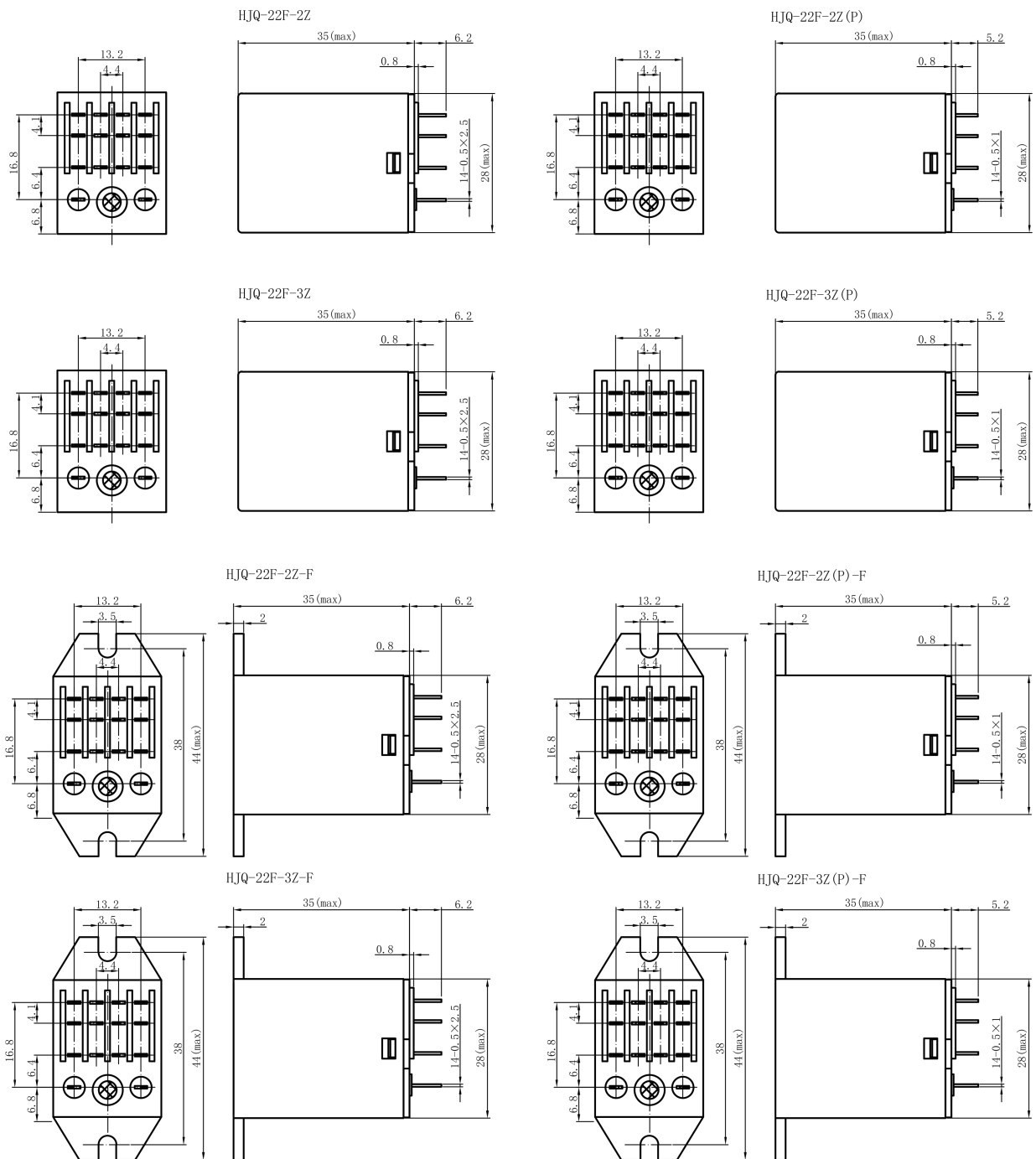
Outline Deminsions 外形图
