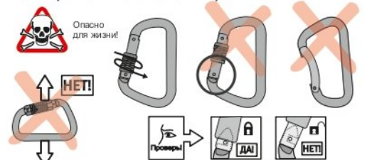
Рис. 7. Ограничения использования карабина
