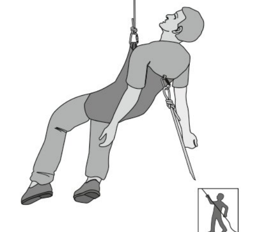
Рис. 9. Спуск и подъем с оттяжкой
