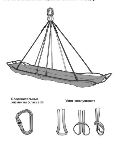
Рис. 3. Использование подвесной системы «Спайдер»
