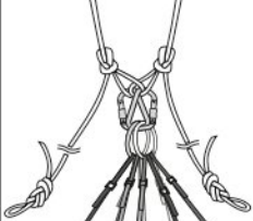
Рис. 5. Способы крепления
