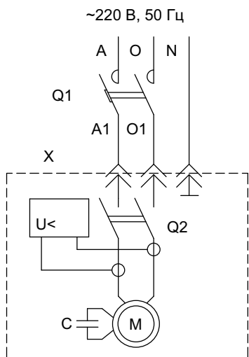
Рис. 3 Схемы электрические.
