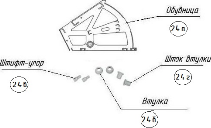
Рис.5 Комплект механизма обувницы
