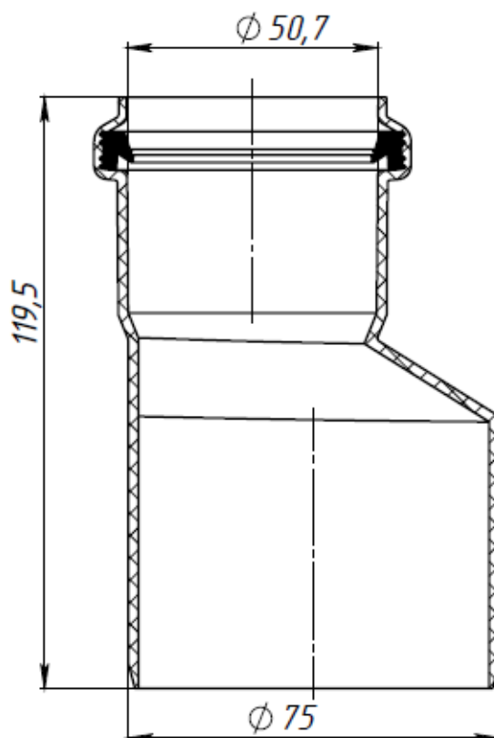
Рис. 1. Схема перехода эксцентрического 75/50
