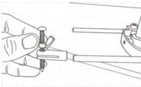
Крепление центра
