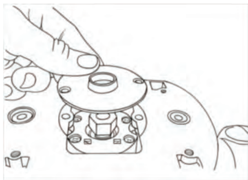
Установка переходной пластины
