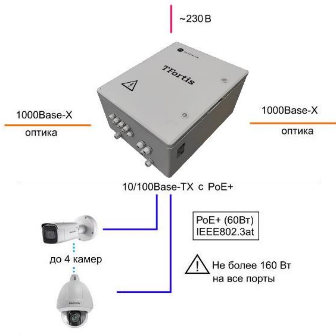
Рисунок 1 - Схема подключения PSW-2G+UPS-Box
