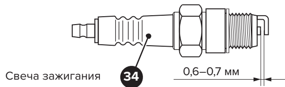
Рисунок 9 — Необходимый зазор в свече зажигания
