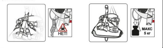
Рис. 18. Способ интеграции рабочего сиденья
