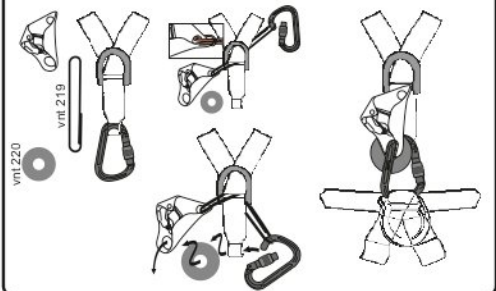
Рис. 13. Соединительно-амортизирующая подсистема
