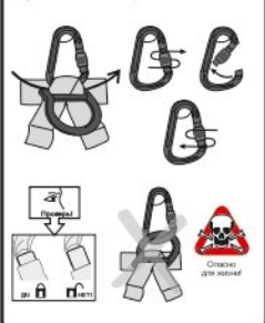
Рис. 12. Страховочная система
