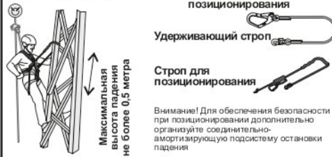
Рис. 17. Пример организации системы канатного доступа
