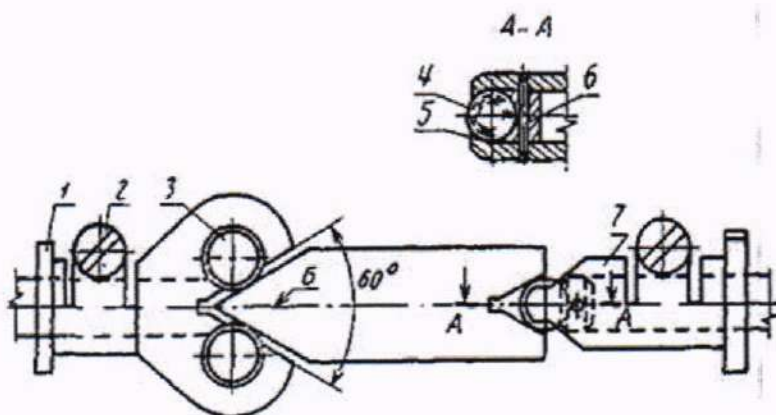
Рисунок 3 – Общий вид специальных наконечников
