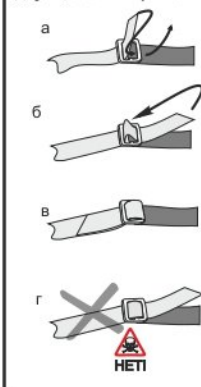
Рис. 4. Использование двухщелевых пряжек
