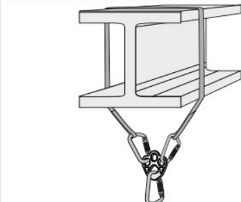
Рис. 3. Использование такелажной пластины
