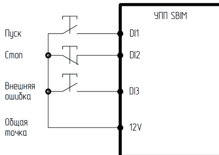
Рис.6. Двух- и трехпроводное подключение
