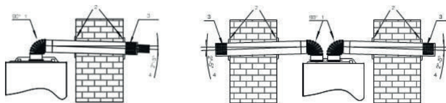
1 - 90° патрубок; 2 - фланец трубы дымохода; 3 - труба дымохода; 4 - уклон 2°-5°
