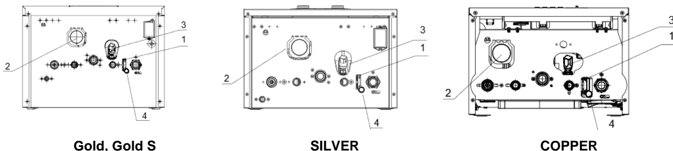
1. Слив предохранительного клапана котла; 2. Манометр; 3. Кран слива котла; 4. Кран подпитки.
