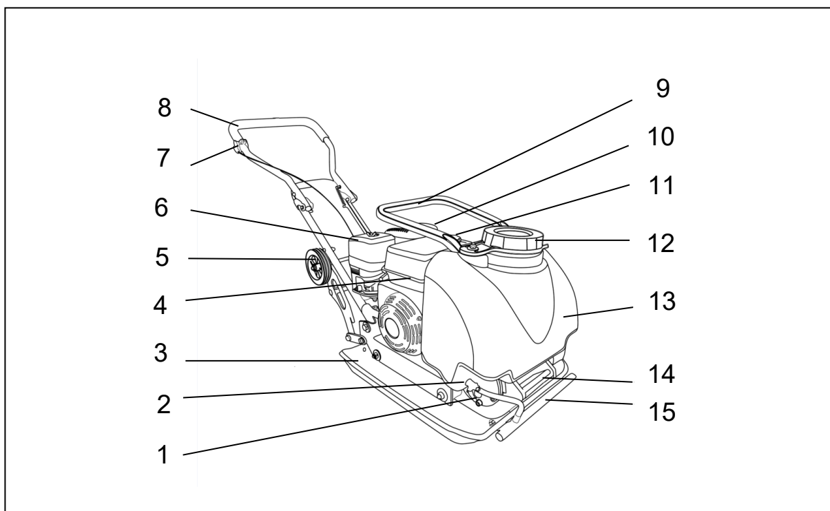
Рис. 1. Общий вид VP-35W, VP-90W, VP-110W
