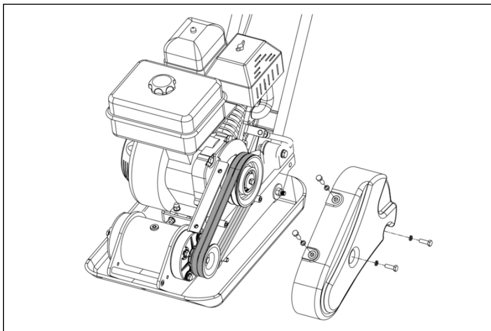
Рис. 20. Проверка состояния ремней.
