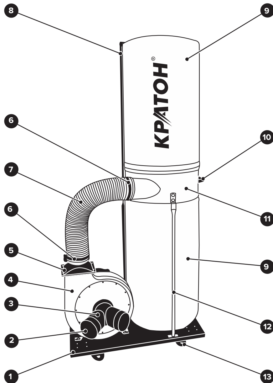
Рисунок 1 — Общий вид пылесоса
