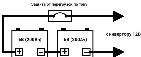
Блок аккумуляторов на 12 В (общая емкость = 200 Ач)
