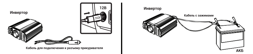
Рисунок 6.1: Подключение инверторов KV-M300/KV-M500/KV-P300/KV-P600
