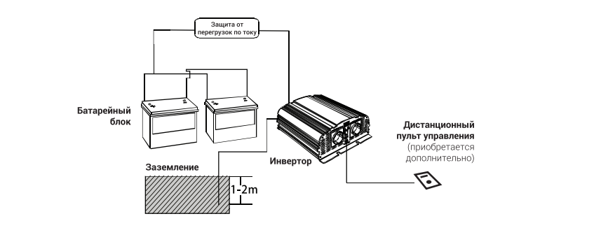
Рисунок 6.2: Подключение инверторов KV-M1000/KV-M1500/KV-M2000/KV-M2500/KV-P1000/KV-P1500/KV-P2000/KV-P3000
