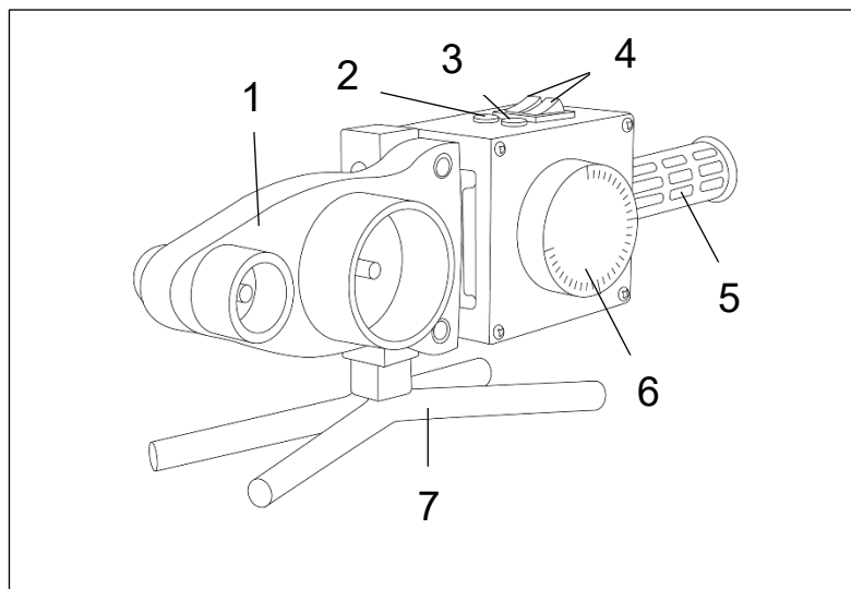
Рис. 1. Общий вид АСПТ- VI72
