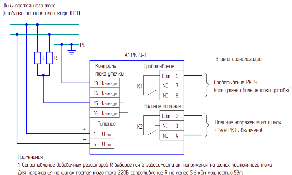
Рисунок ПЗ.1. Схема подключения реле «РКТУ-1» для контроля тока утечки в цепи постоянного тока
