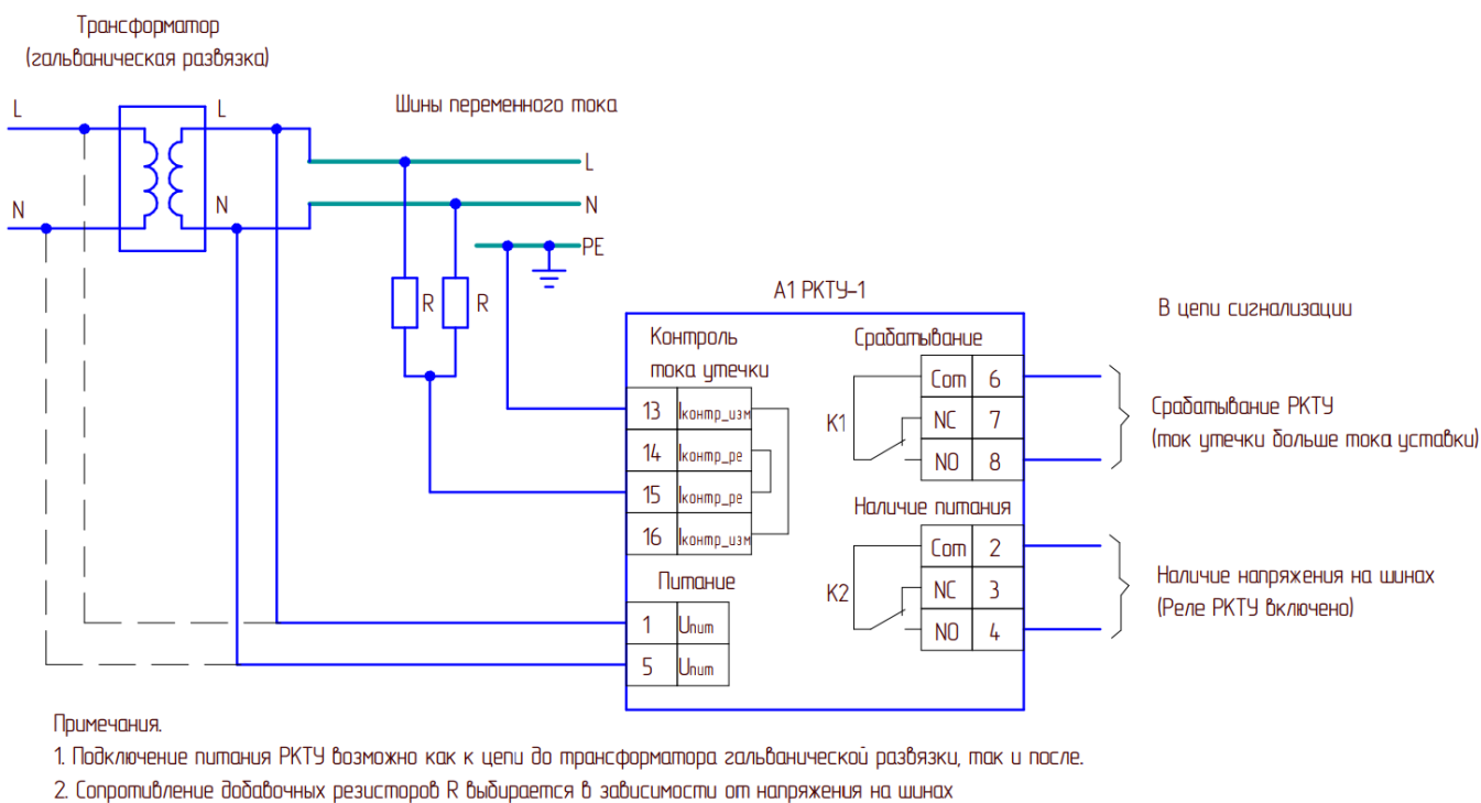
Рисунок ПЗ.2. Схема подключения реле «РКТУ-1» для контроля тока утечки в цепи переменного тока
