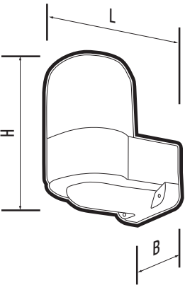
Рис.1 Светильник PWL
