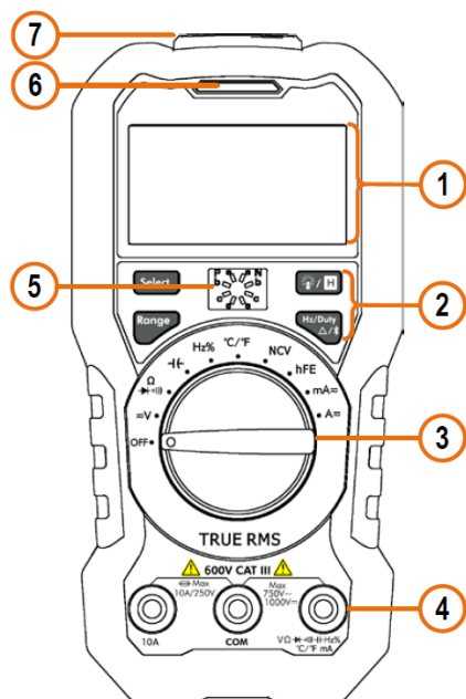
Рисунок. 2.1. Общий вид передней панели (на примере модели OW16B с функцией тестирования транзисторов)
