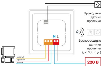
Шаровые краны с электроприводом Ujin Aqua-drive
