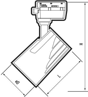
Рис 1. Прожектор PTR 17
