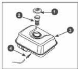
Рис. 26 Топливные фильтры
