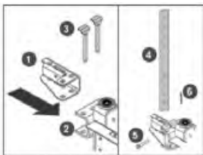
Рис. 4 Установка сошника
