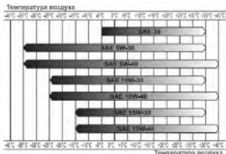
Рис. 10 Определение вязкости масла
