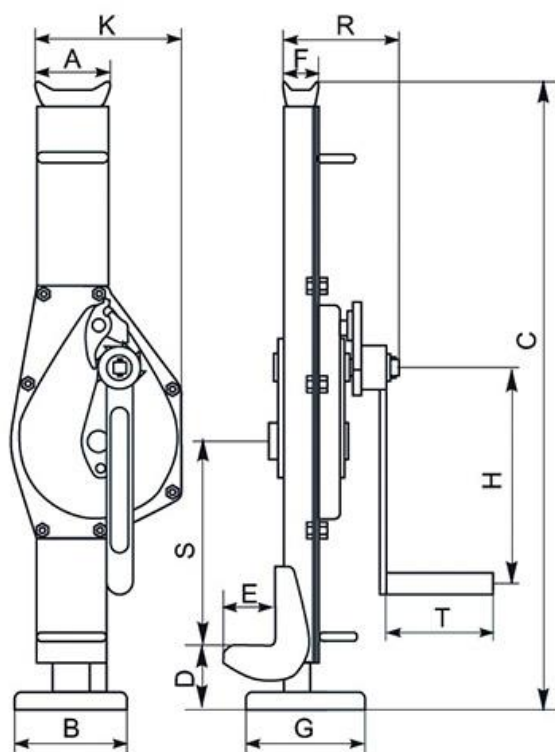
Рисунок 1 Размеры домкрата
