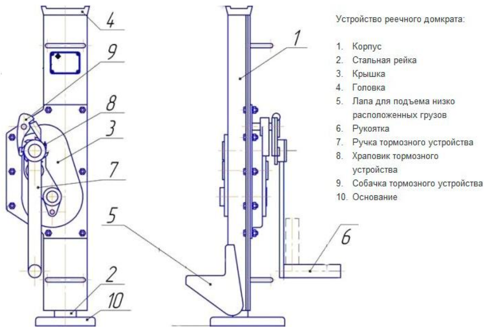
Рисунок 2 Устройство домкрата
