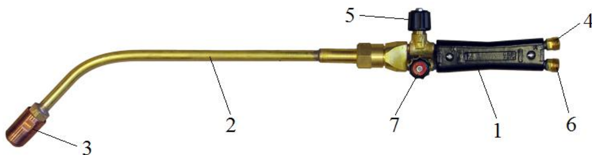
Рис.1. Горелка ГП-1 Вулкан
