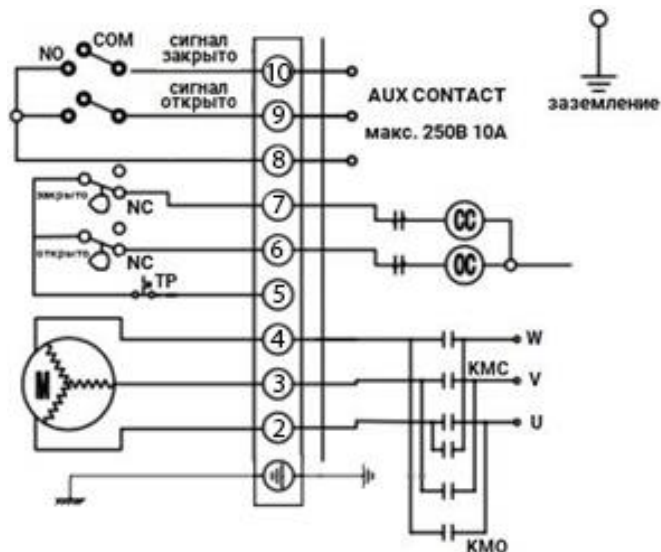
Рисунок 4 – Схема подключения на 380 В
