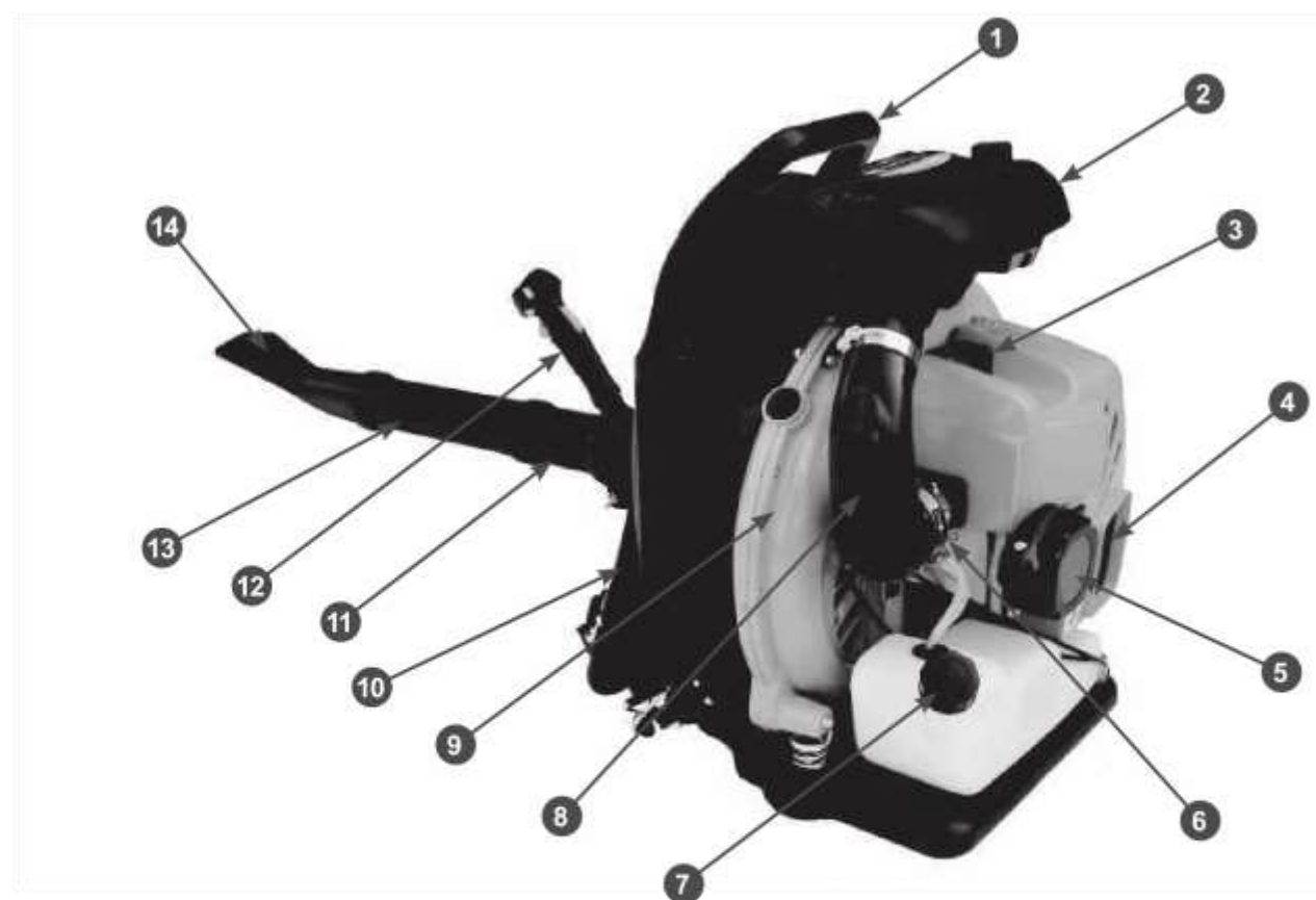
Рис. 1 Основные узлы и органы управления
