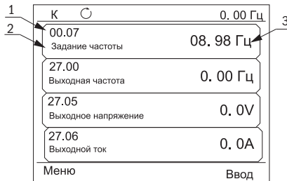
Рисунок 4.16 – Выбор параметра монитора состояния
