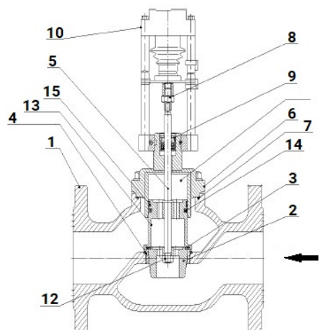
Разгруженный по давлению клапан DN50 – 100. Исполнение Б.
