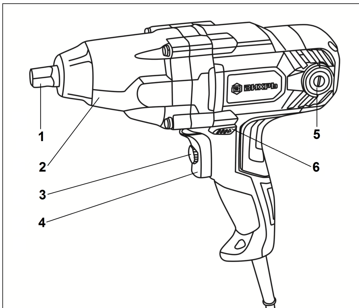
Рис.1. Общий вид.
