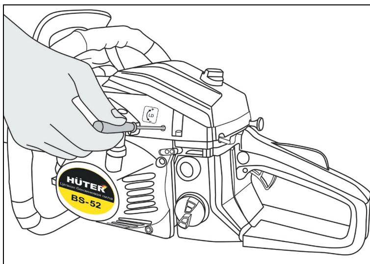
Рис.40 Регулировка оборотов
