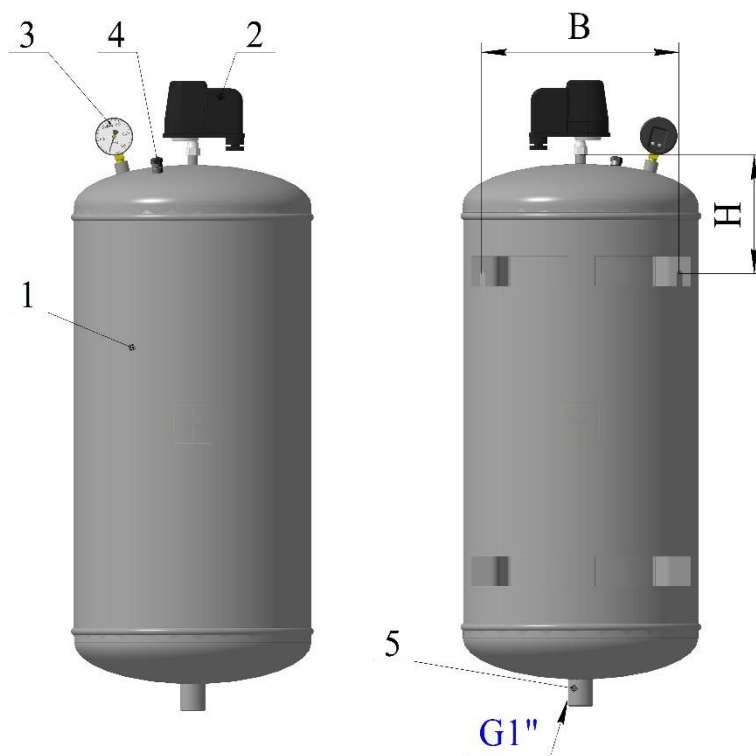
Гидроаккумулятор настенный
