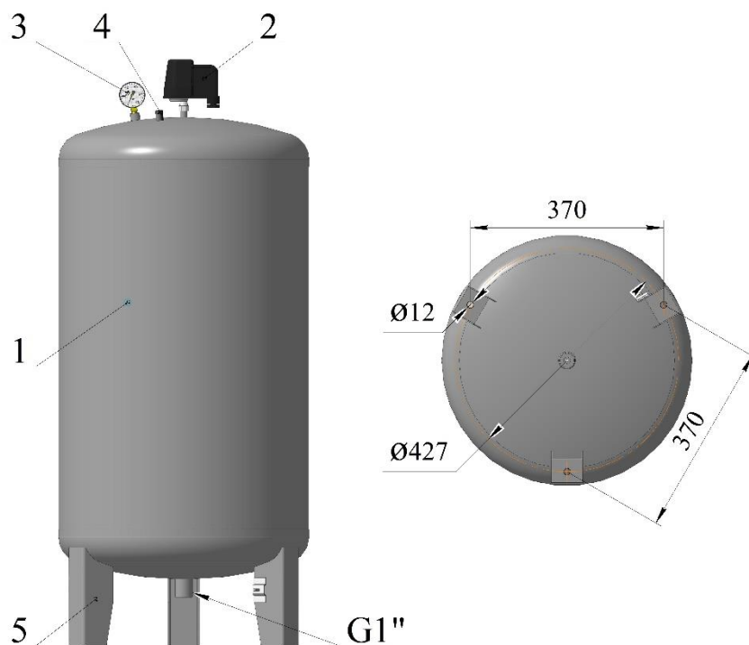
Гидроаккумулятор напольный
