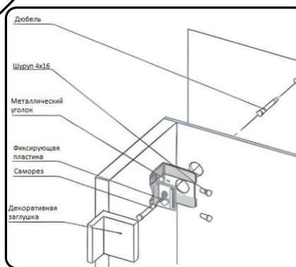
Крепление навеса шкафа
