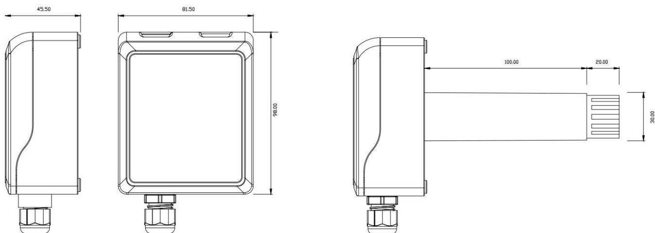
Рис.1. Габаритные размеры канальных датчиков
