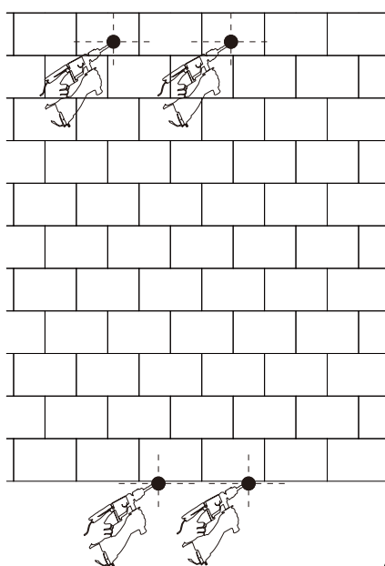
Сделать отверстия D 10 mm глубиной 50 mm
