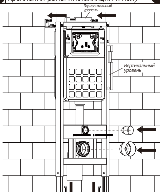
Зафиксировать раму инсталляции к полу и стене
