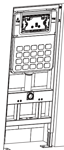
Монтаж полностью в фальшстену
