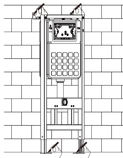
Вывести по вертикали и горизонтали, сделать разметку под отверстия крепления рамы инсталляции к полу
