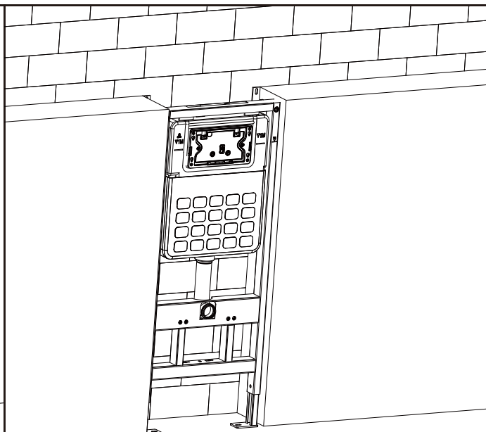
Монтаж в фальшстену по высоте рамы инсталляции
