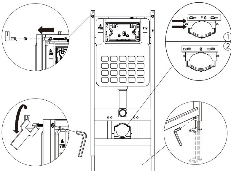
Монтаж полностью в фальшстену
