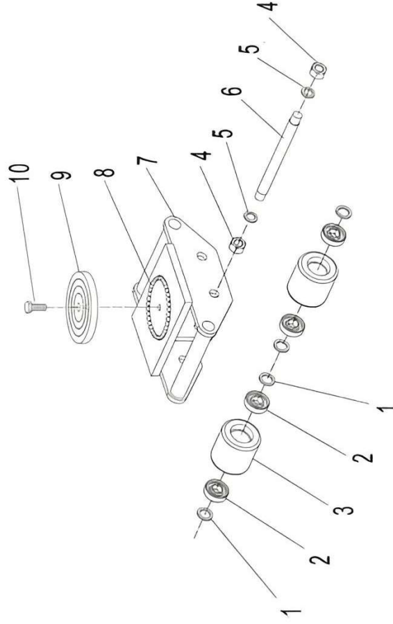
Рисунок 4 – Взрыв-схема роликовой платформы CRA 4.
