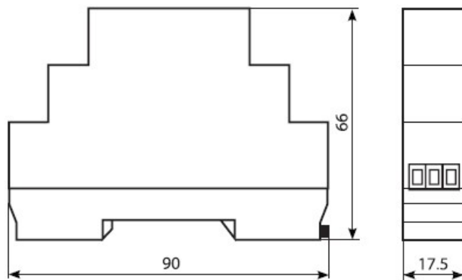
Рис2. Размеры корпуса.
