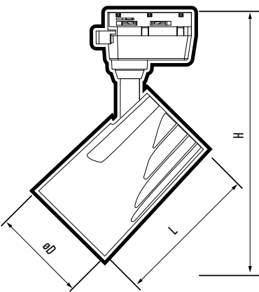
Рис 1. Прожектор PTR 17
