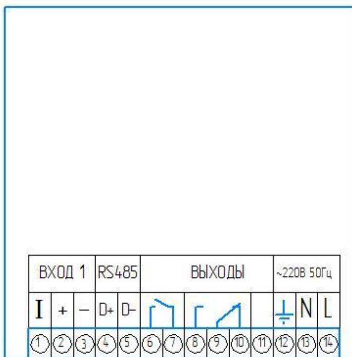
Схема расположения и состав выходов ИСУ101
