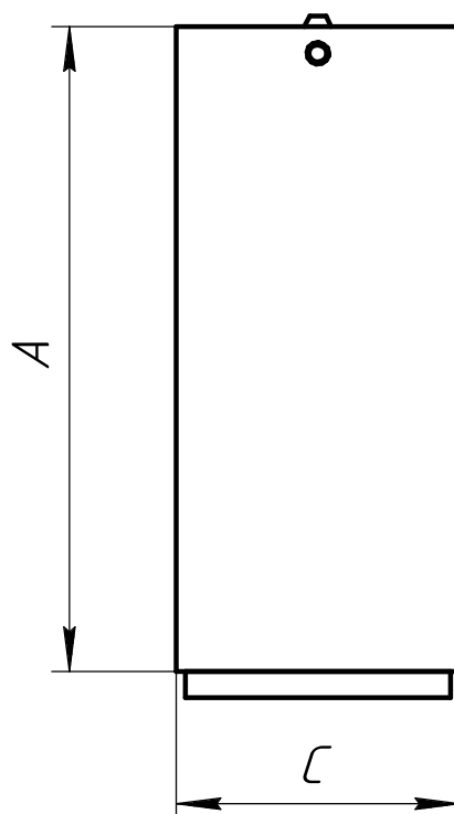
Рисунок 1 - Общий вид, габаритные размеры светильника ДПО28.
