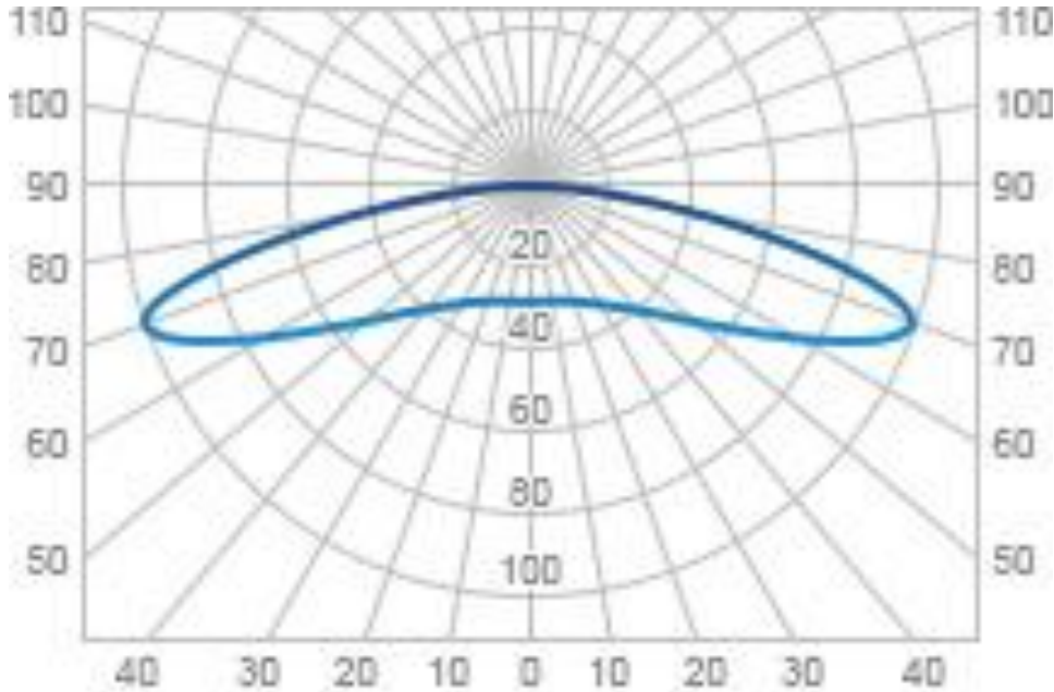
Рисунок 3 тип КСС в исполнении "Ш"
