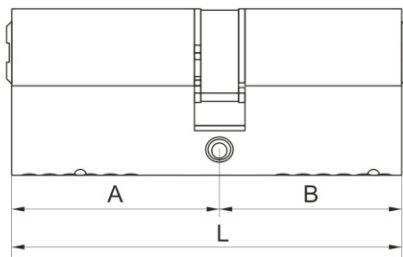
Ключ-ключ
