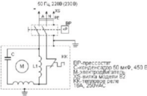
Схема электрическая принципиальная модели: OPT-302430, OPT-305030
