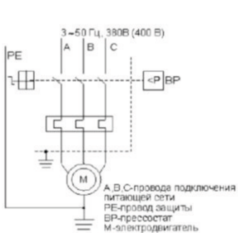
Схема электрическая принципиальная модель OPT-301042
