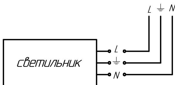
Рисунок 4 - Схема подключения светильников к сети
